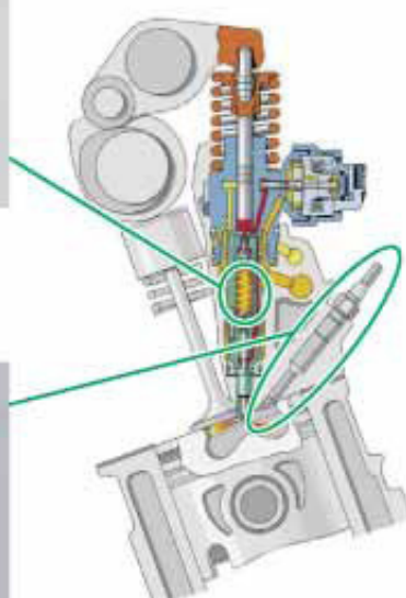
ディーゼルエンジンの断面図
