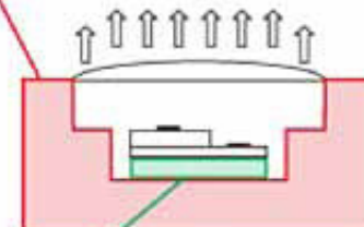
LED構造図
