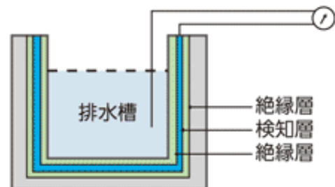
漏洩検知システム
